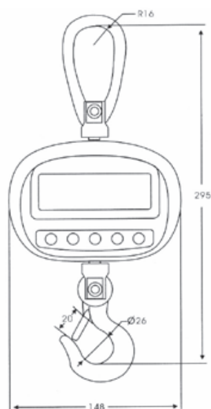
Fig. 1 unité : mm
