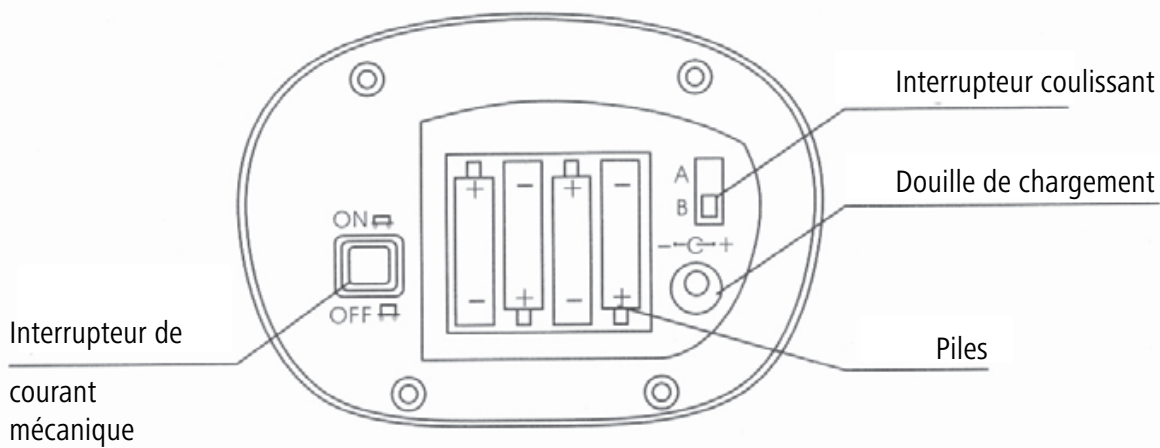
Fig. 3 Schéma du l'arrière du boîtier du peseur
